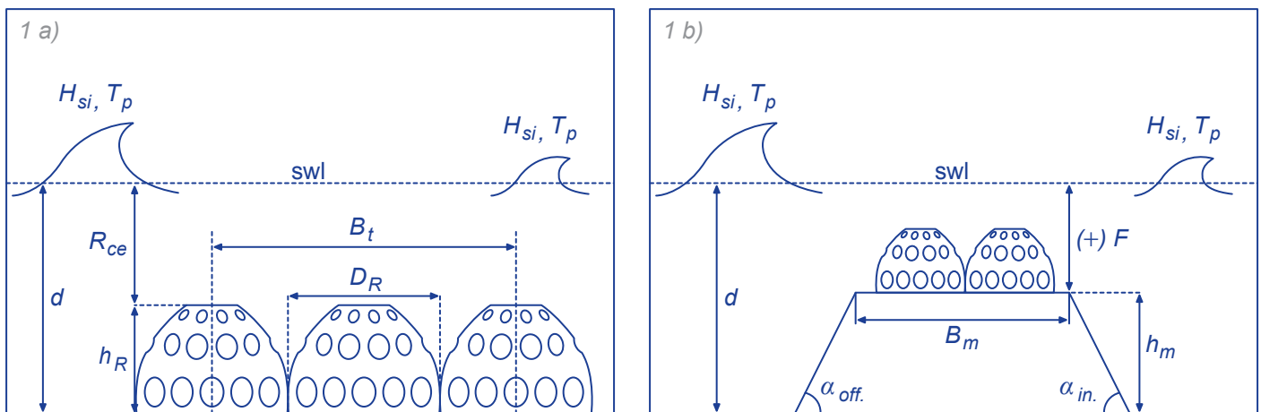
Figura 1 – Schema delle variabili adoperate in caso di elementi Reef Ball posizionati (a) direttamente sul fondale (b) sulla cresta di una gettata tradizionale
